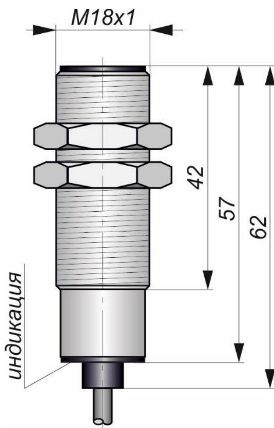
Габаритный чертеж
