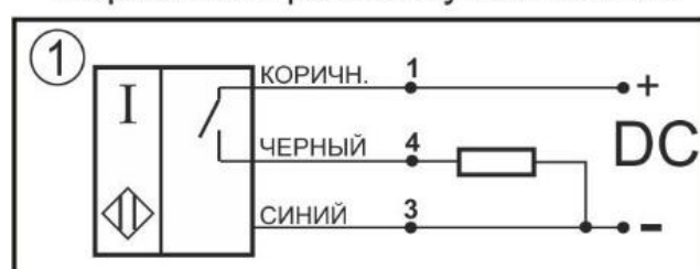
Нормально-разомкнутый контакт
